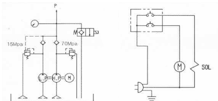
HEP103241LS AN HEP103242LS CIRCUITS
