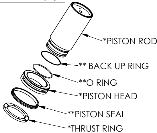
FIG1 2 PART PISTON
