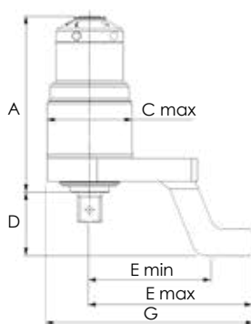
NTM40, NTM70
