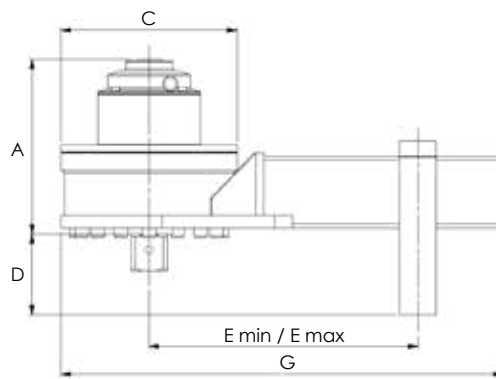
NTM95
