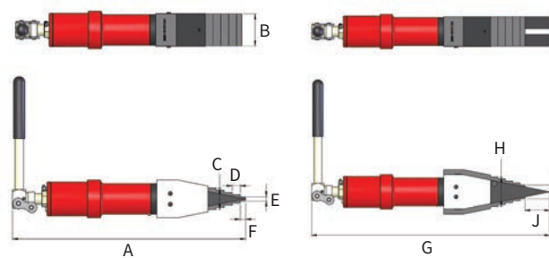
SJS10-M回缩
